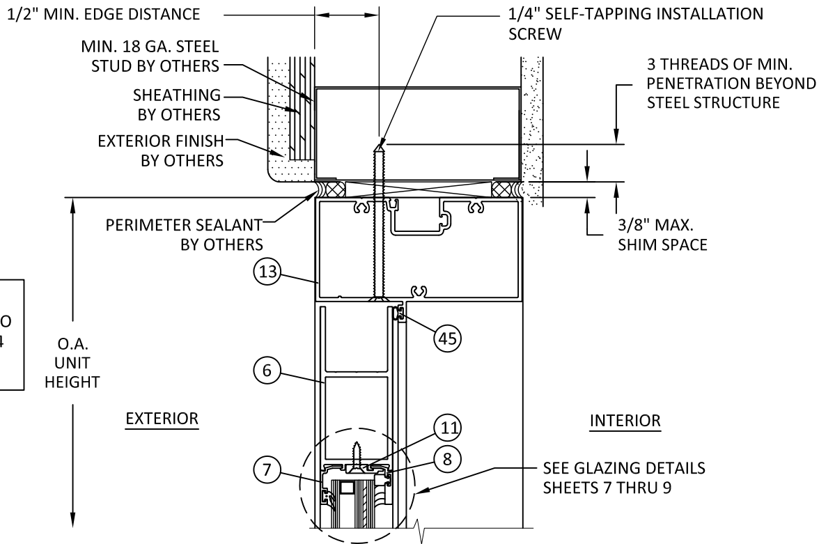
C 3 VERTICAL SECTION DOOR HEAD - STEEL STUD
