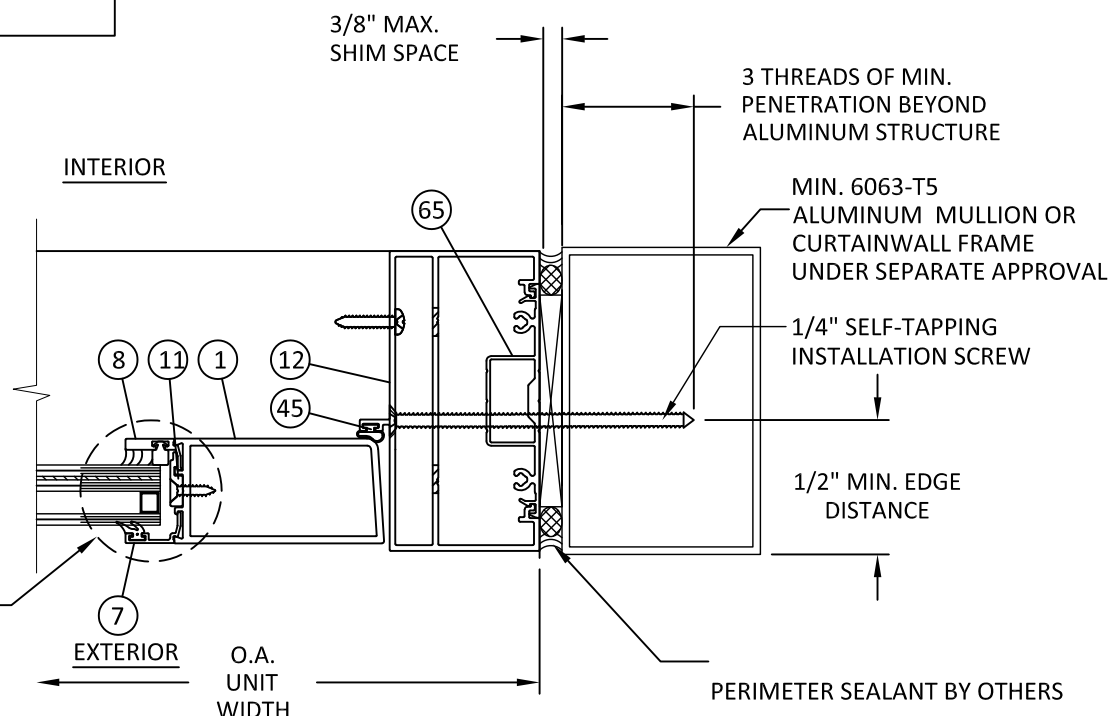
H HORIZONTAL SECTION 4 DOOR JAMB - ALUMINUM STUD
