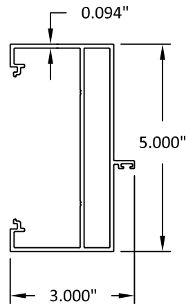
DOOR JAMB
